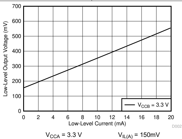
图 6-3. 低电平输出电压 ( V_{OL(Ax)} ) 与低电平电流 ( I_{OL(Ax)} ) 间的关系
