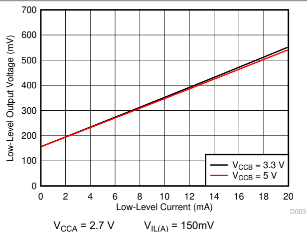
图 6-2. 低电平输出电压 ( V_{OL(Ax)} ) 与低电平电流 ( I_{OL(Ax)} ) 间的关系
