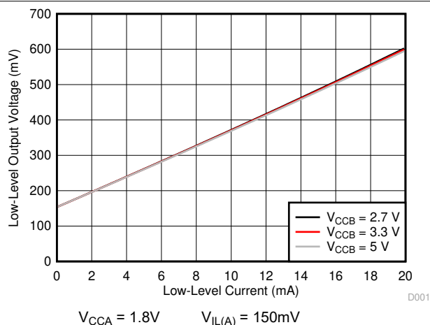
图 6-1. 低电平输出电压 ( V_{OL(Ax)} ) 与低电平电流 ( I_{OL(Ax)} ) 间的关系
