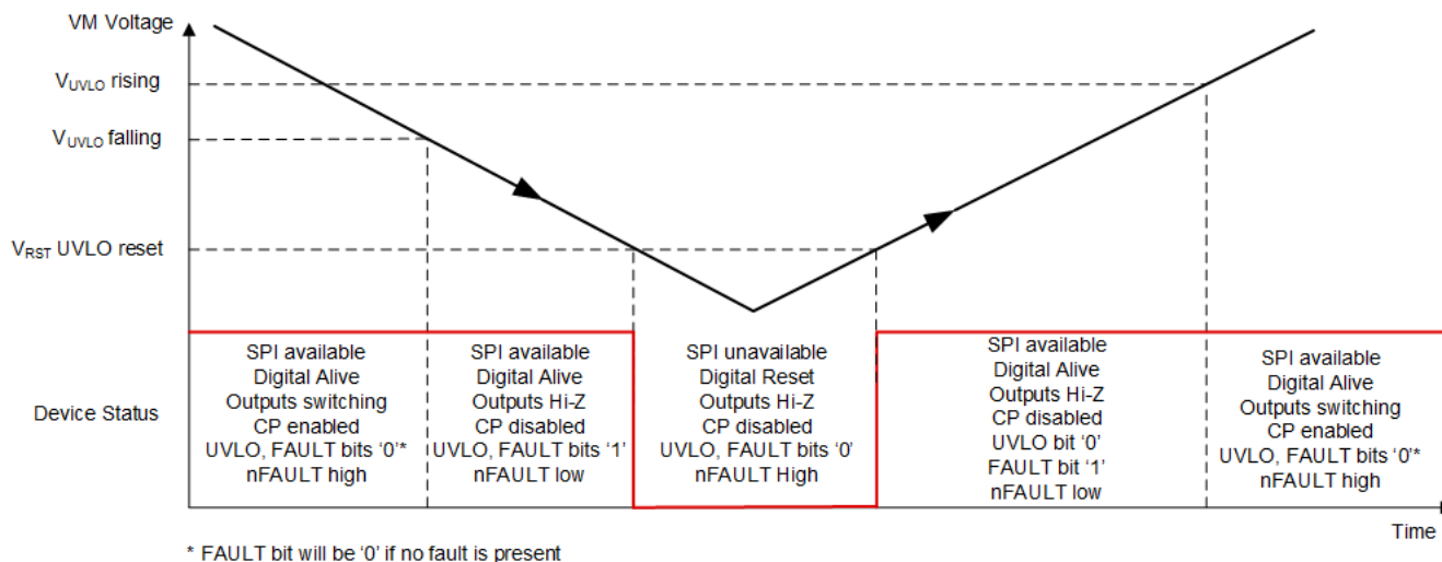
图 7-20. 电源电压斜坡曲线
