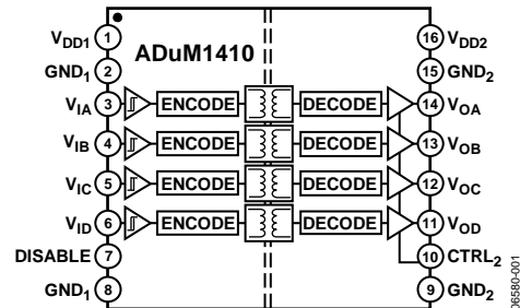
图1. ADuM1410
