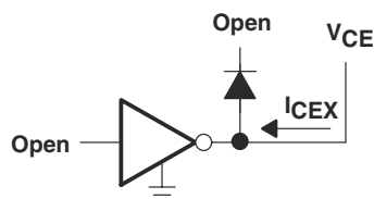
图 7-1. I_{CEX} 测试电路
