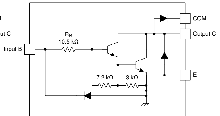
图 8-3. ULN2004A 和 ULQ2004A 方框图
