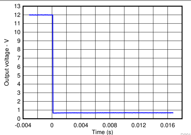
图 9-2. 线圈激活时的输出响应 ( 接通 )
