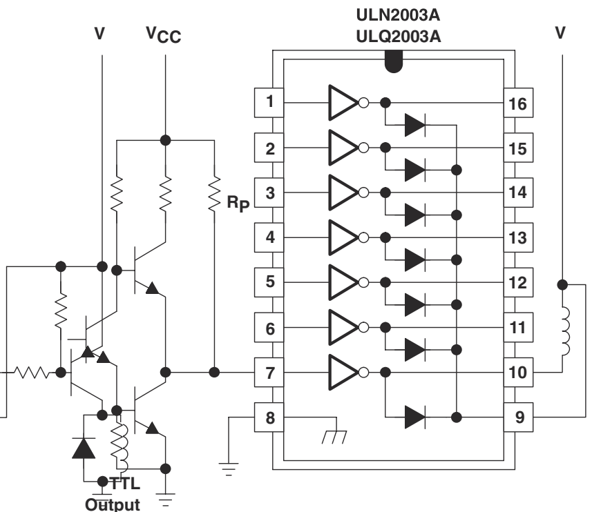
图 9-7. 使用上拉电阻来增加驱动电流
