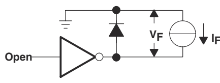
图 7-8. V_F 测试电路
