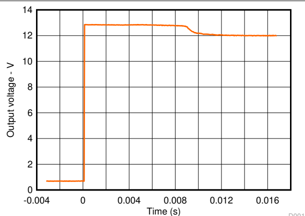
图 9-3. 线圈去激活时的输出响应 ( 关断 )
