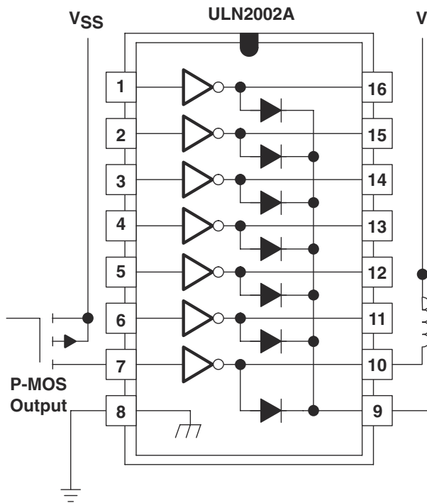
图 9-4. P-MOS 到负载
