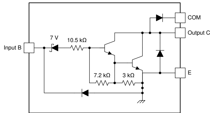
图 8-1. ULN2002A 方框图
