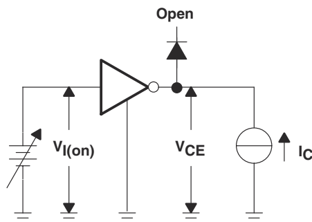
图 7-6. V_{I(on)} 测试电路
