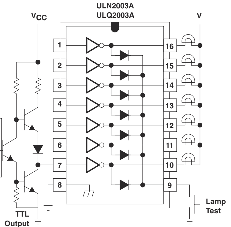
图 9-5. TTL 到负载
